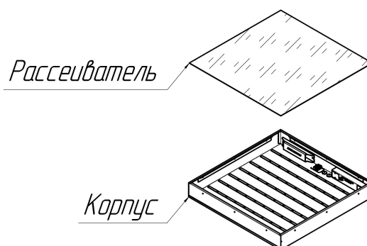
Рис. 2 Взрыв-схема.
