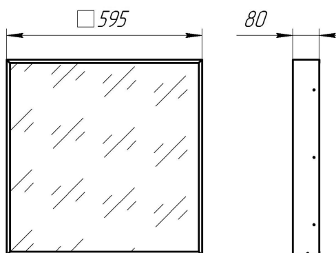
Рис. 1 Габаритный чертеж
