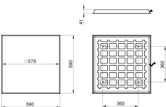
Рис.1 Габаритный чертёж.
