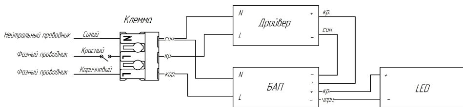
Рис. 3 Схема подключения.
