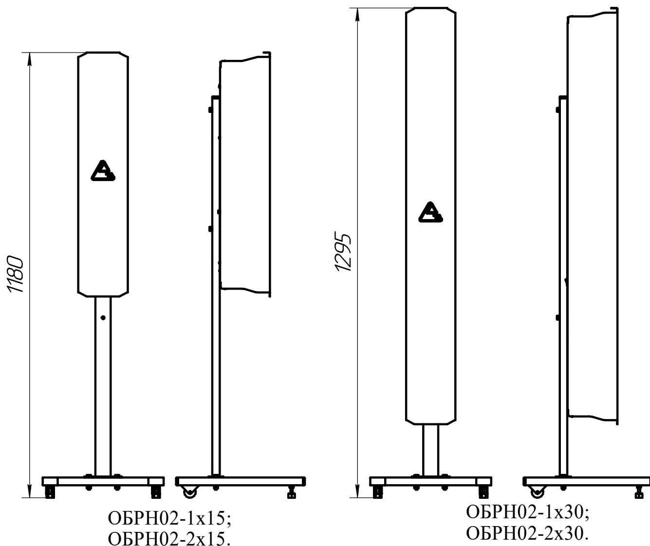
Рисунок 2. Стойка передвижная с установленным рециркулятором (рециркулятор в комплект поставки не входит)
