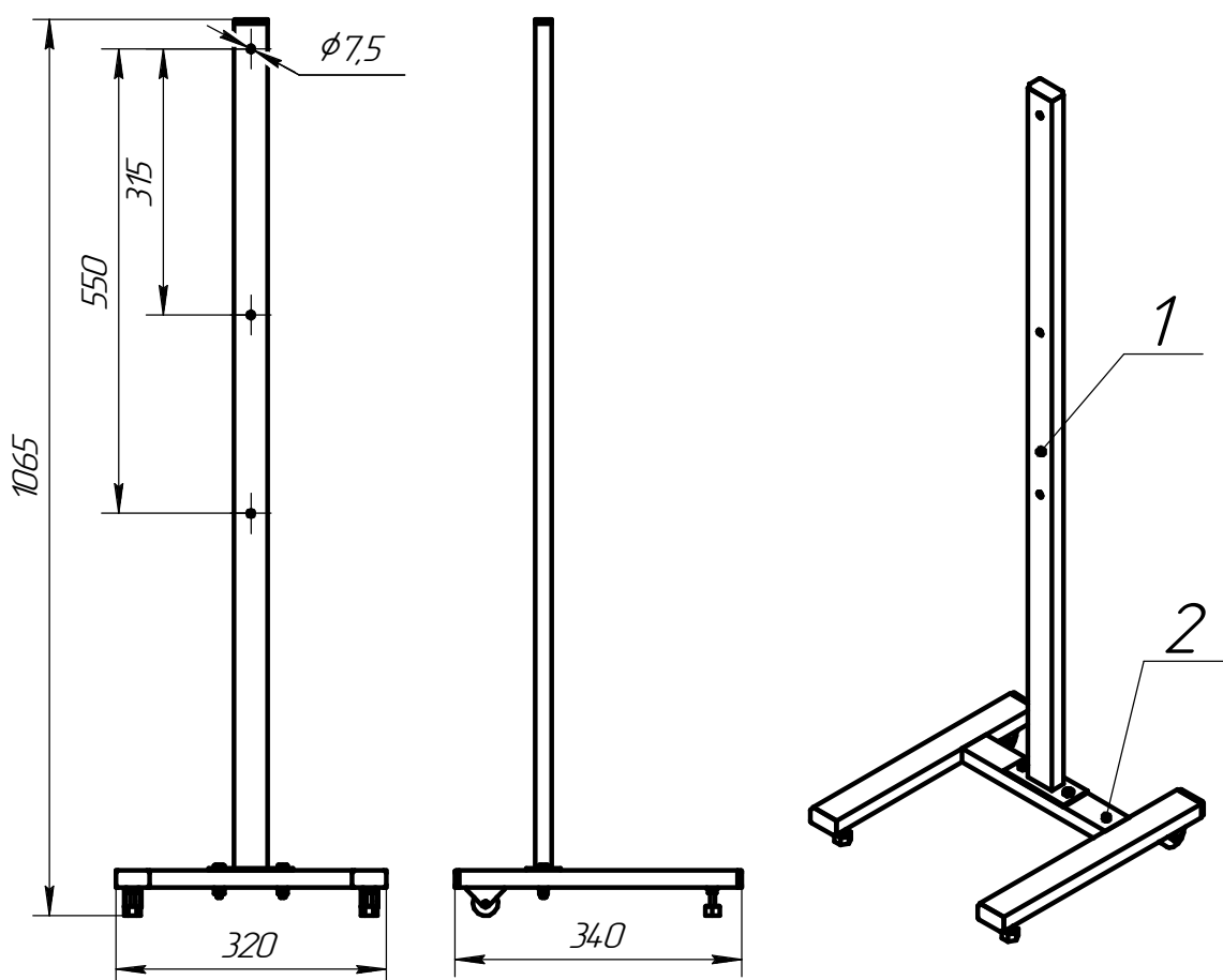
Рисунок 1. Стойка в сборе.
