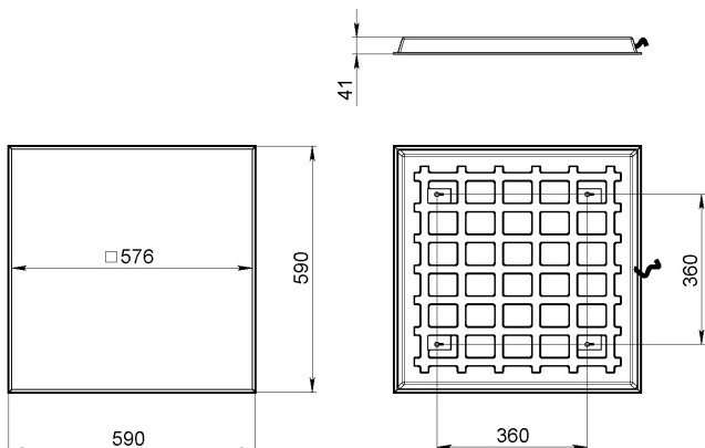
Рис.1 Габаритный чертеж.
