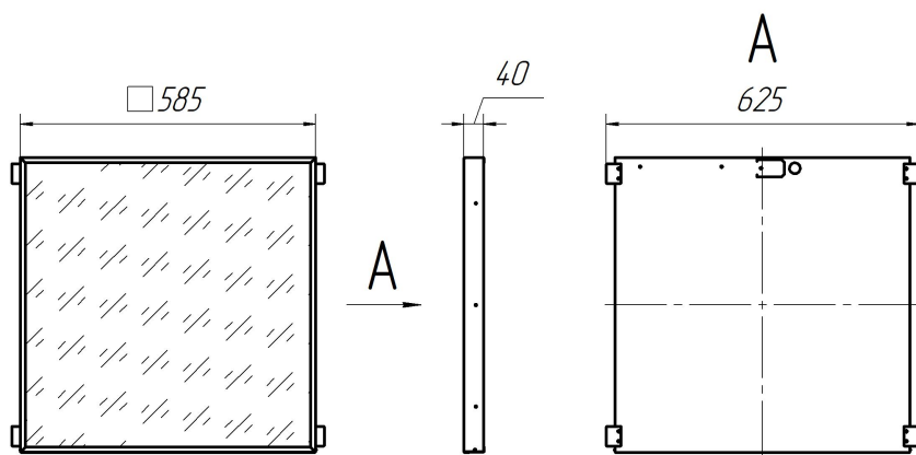
Рис. 1 Габаритный чертеж.
