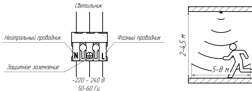
Рис. 2 Схема подключения.
