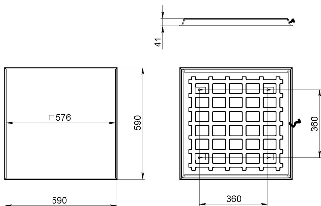
Рис.1 Габаритный чертеж.
