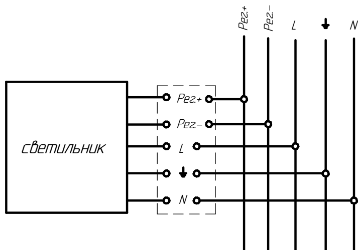
Рисунок 5 - Схема подключения светильника с управлением к сети
