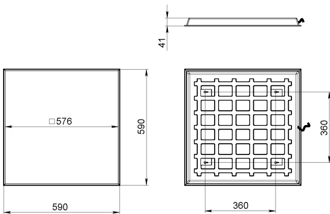
Рис.1 Габаритный чертёж.
