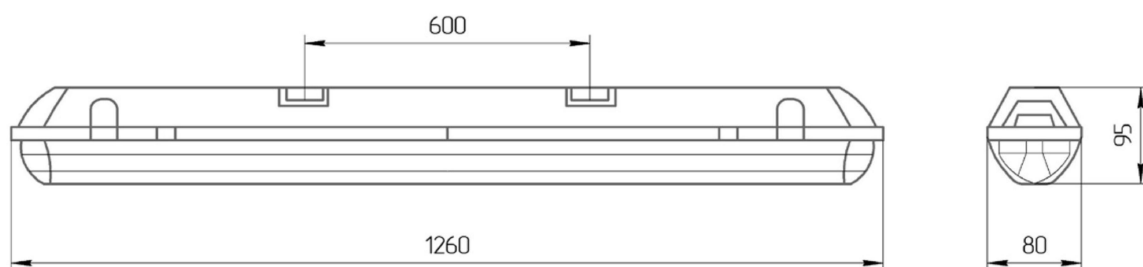
Рис. 1 Габаритный чертеж.
