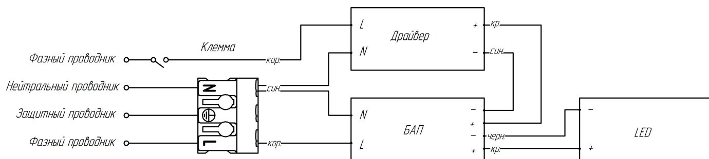
Рис. 2 Схема подключения.
