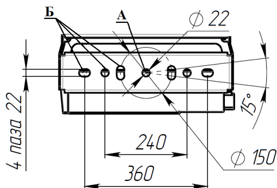
Монтажные отверстия
