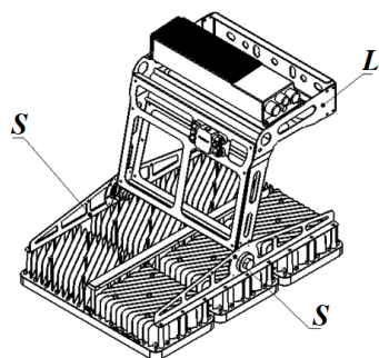
Переноска прожектора
