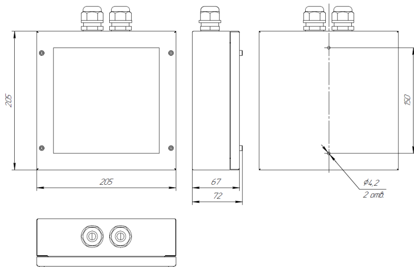
Рис. №2 Габаритный чертёж.
