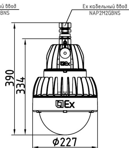
Globus LED D270 G Ex
