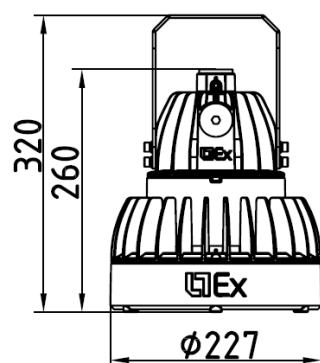
Globus LED D120 B Ex
