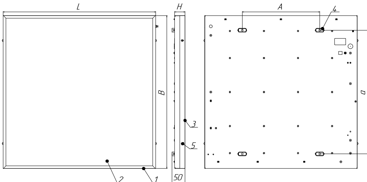
Рисунок 1 - Светильник Alenka LED/S 1 - корпус, 2 - рассеиватель, 3 - боковая планка, 4 - проставка пластиковая, 5 - винт.
