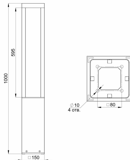
Габаритный чертеж
