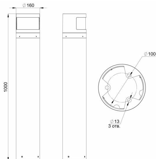
Габаритный чертеж
