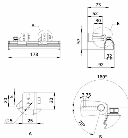
Габаритный чертеж
